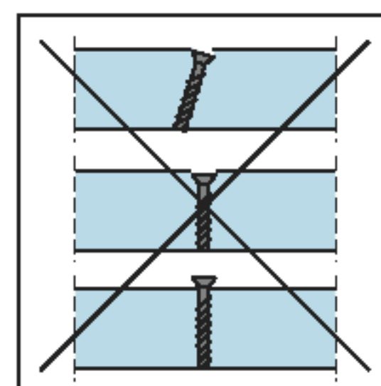
Неправильная установка шурупа
