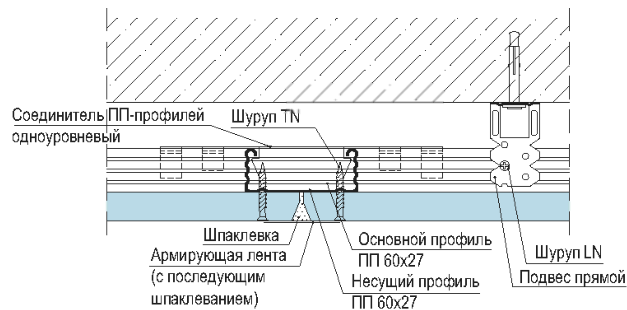
Г - Г Присоединение основных профилей
