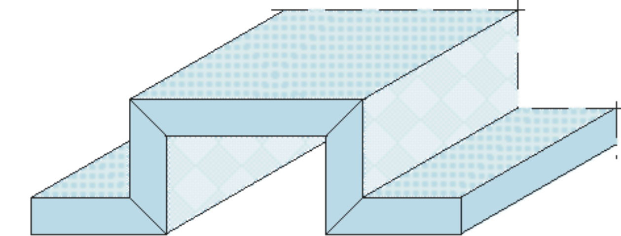
3 x 90° V-вырезы
