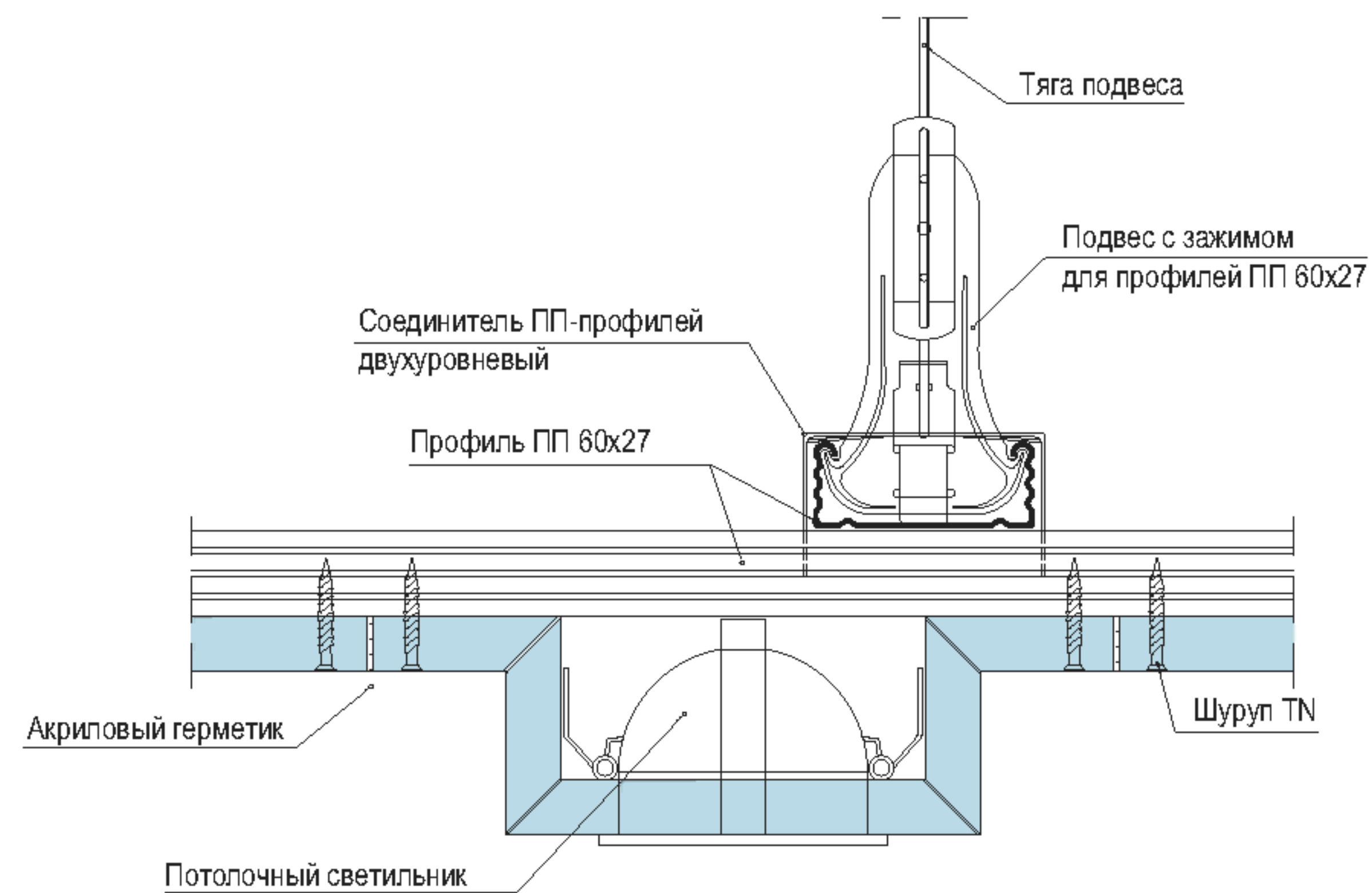
Выпуклый потолок со светильником
