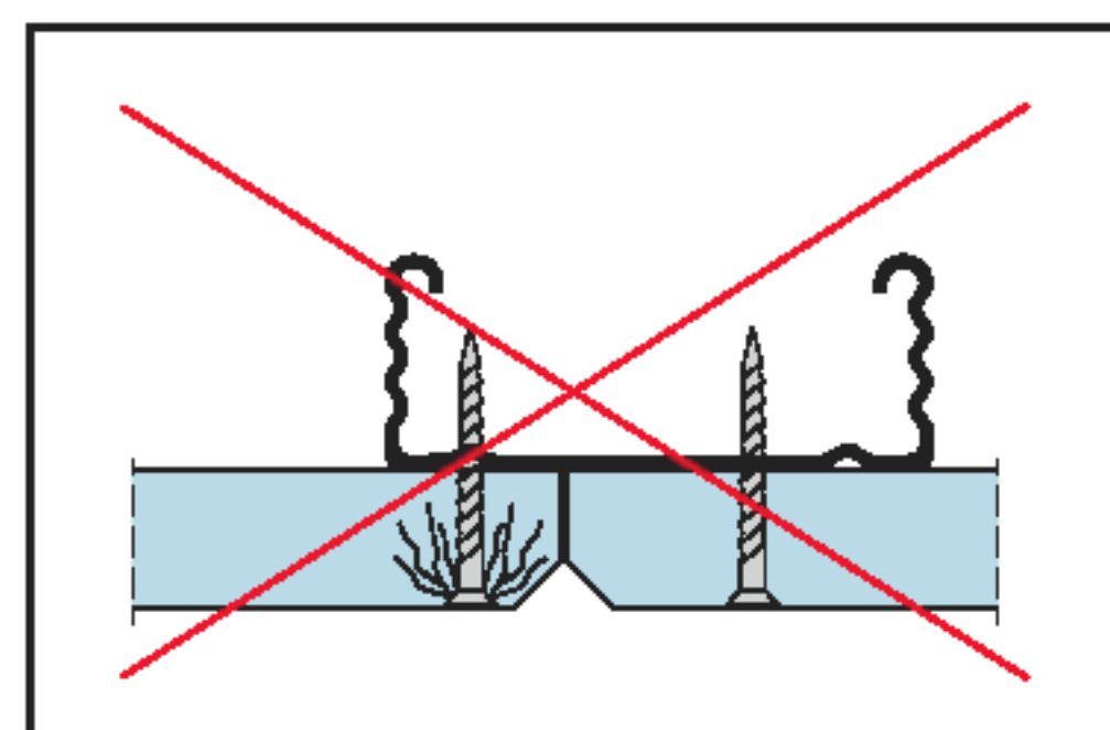
Неправильное крепление к профилю гипсокартонного листа
