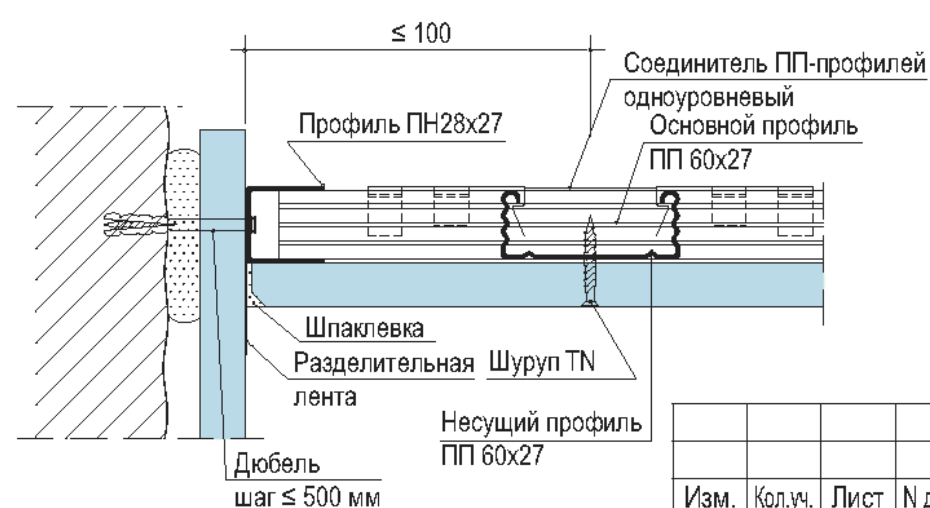
Б - Б Примыкание к стене
