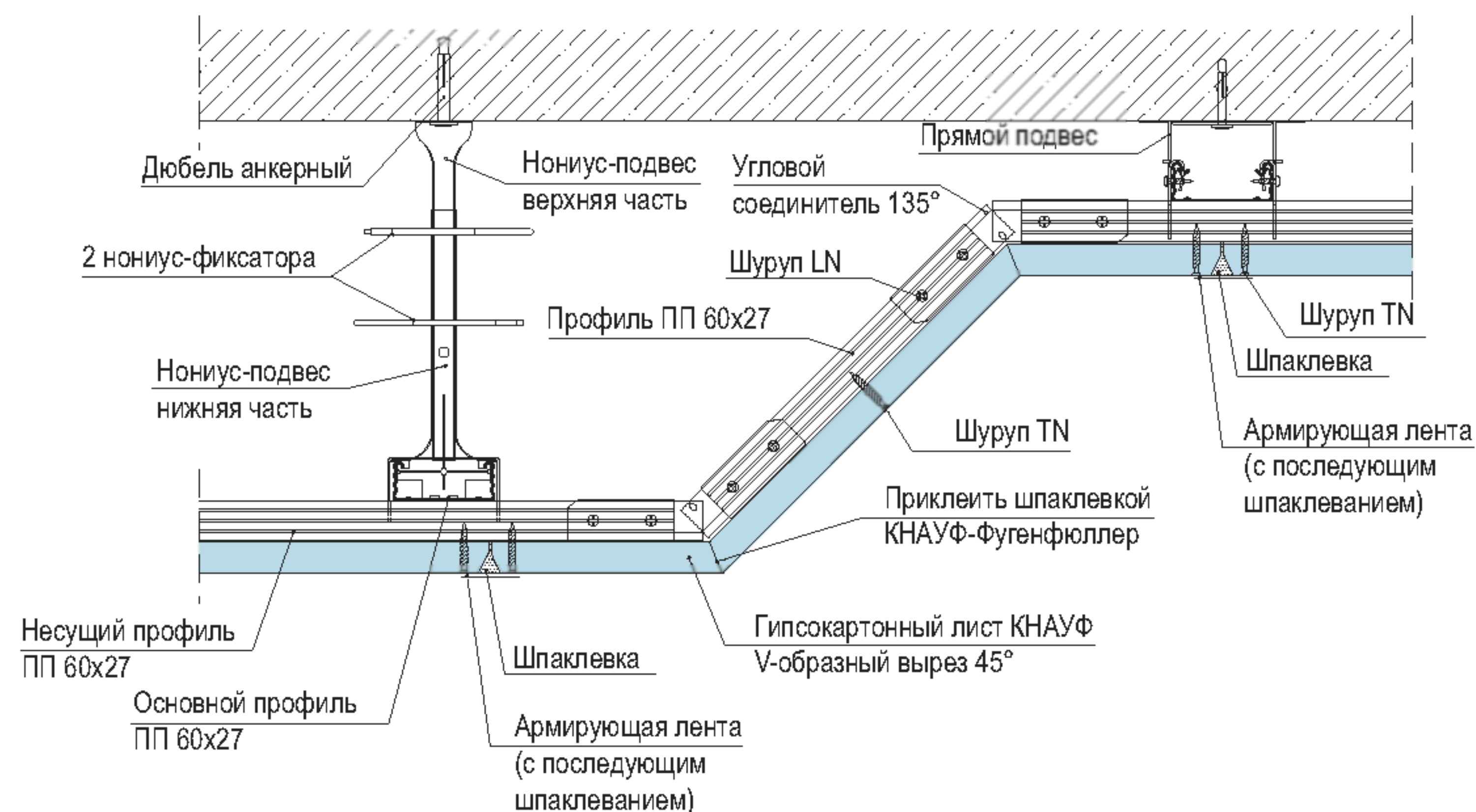
Угловой соединитель
