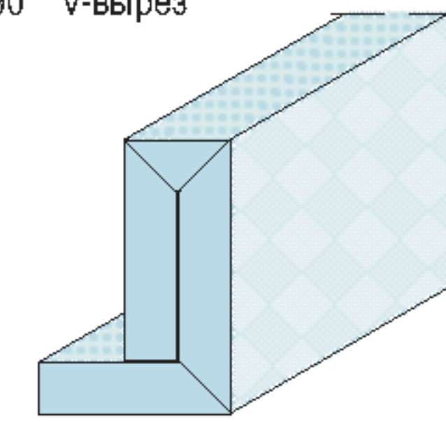
1 x 90° V-вырез
