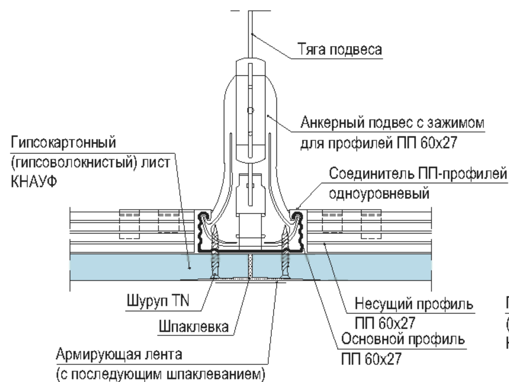
Г - Г Присоединение основных профилей
