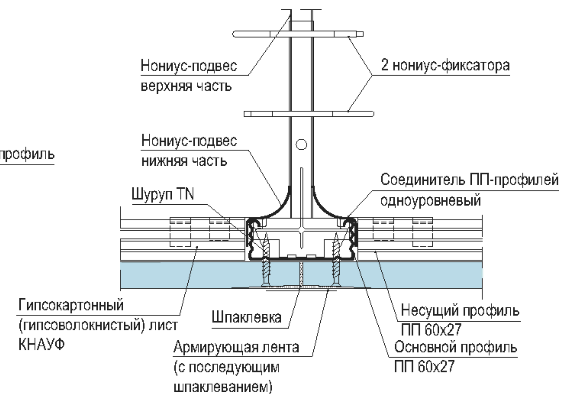
Г - Г Присоединение основных профилей
