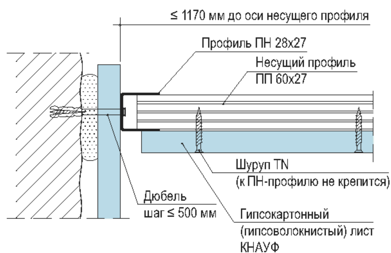
А - А Примыкание к стене видимым швом
