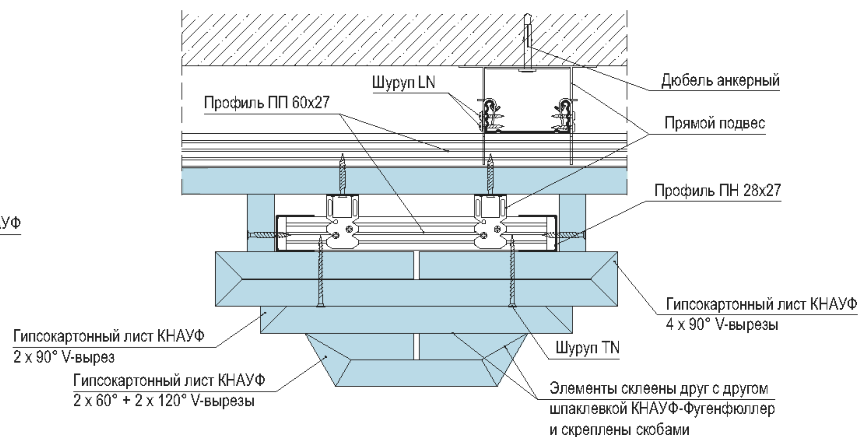
Пример применения - потолочный блок - ступенчатое расположение
