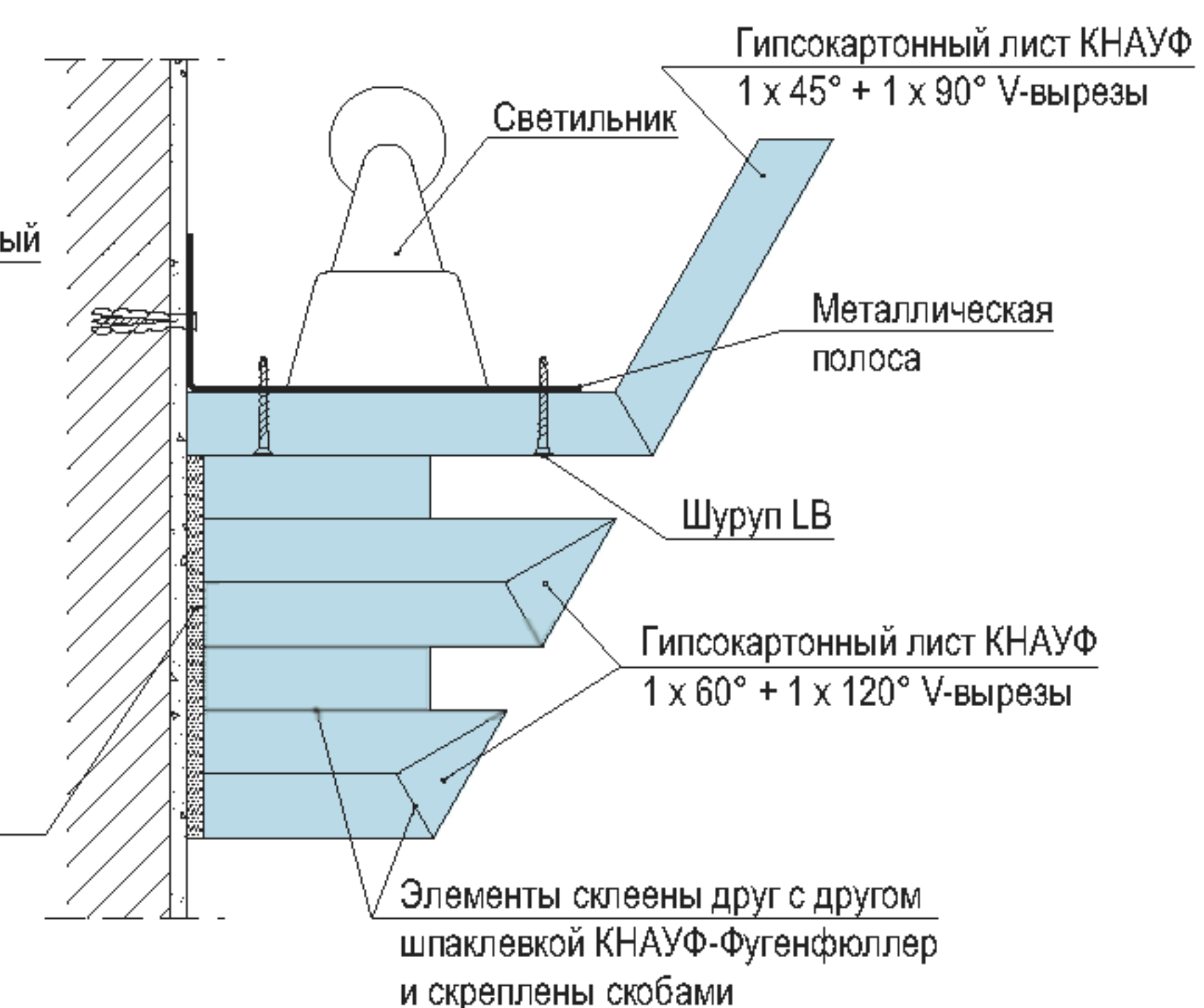
Пример применения - карниз для непрямого освещения
