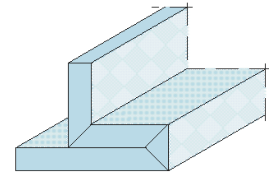
2+2 x 90° V-вырезы
