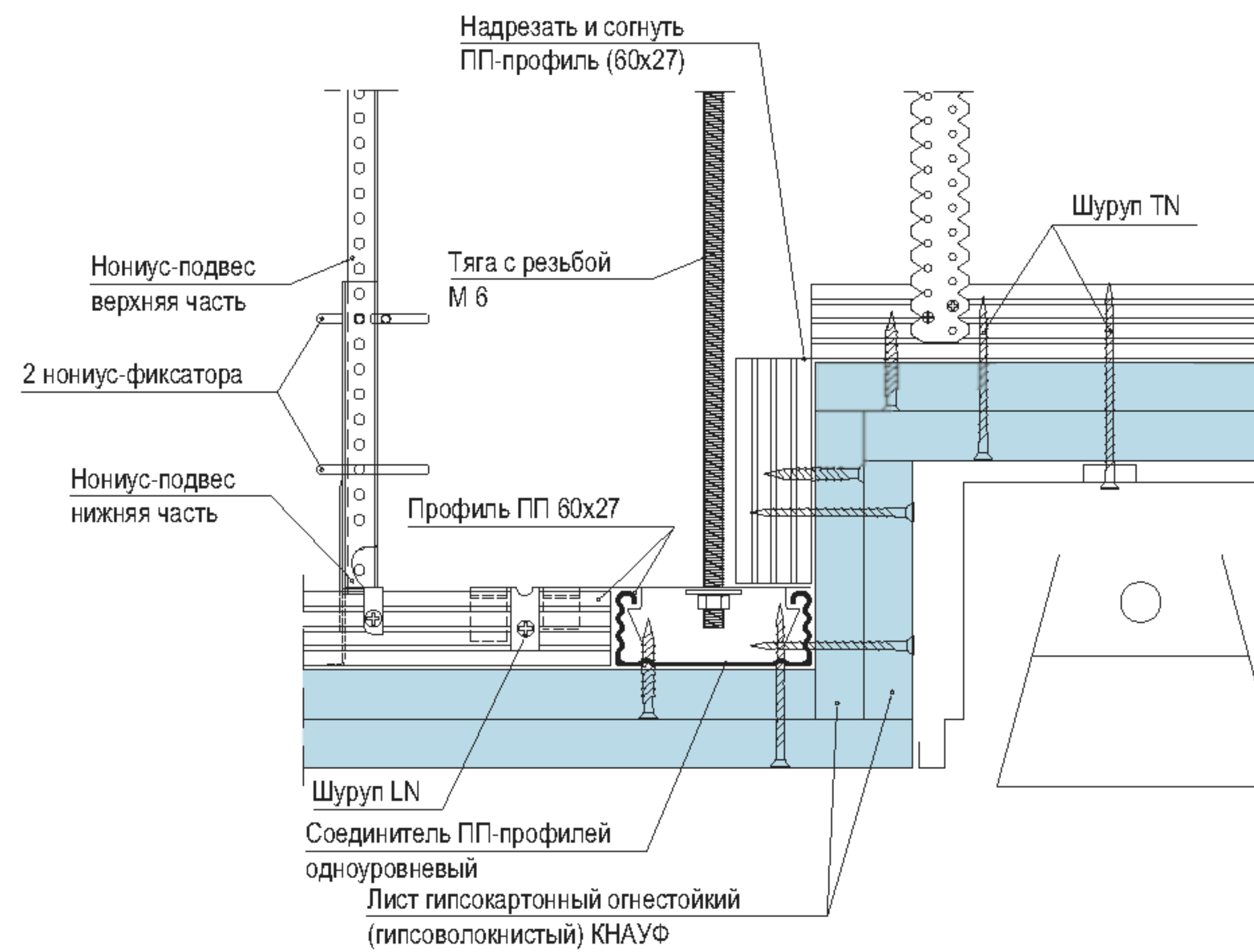
Выпуклый потолок со светильником
