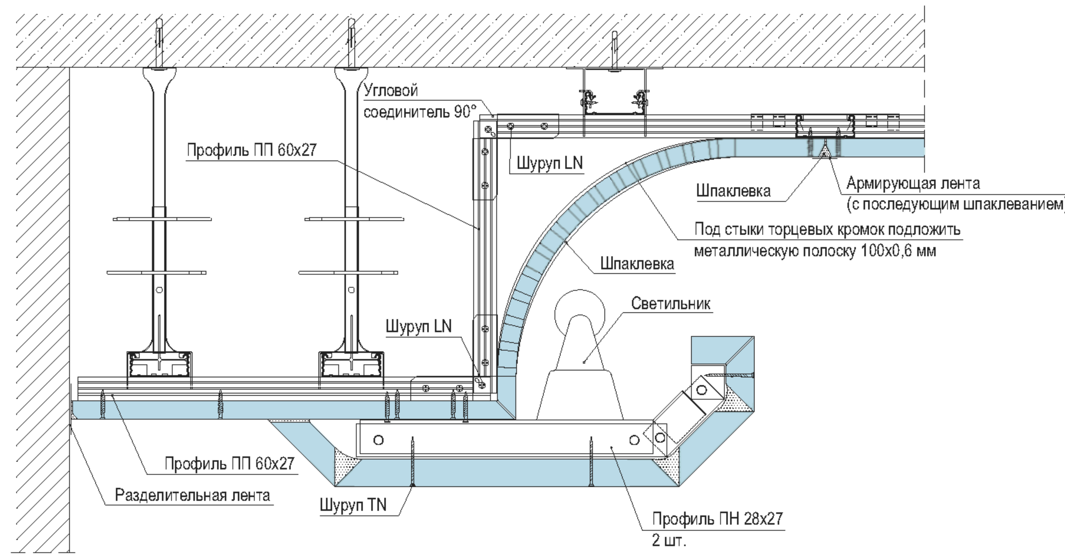
Пример применения – световая падуга
