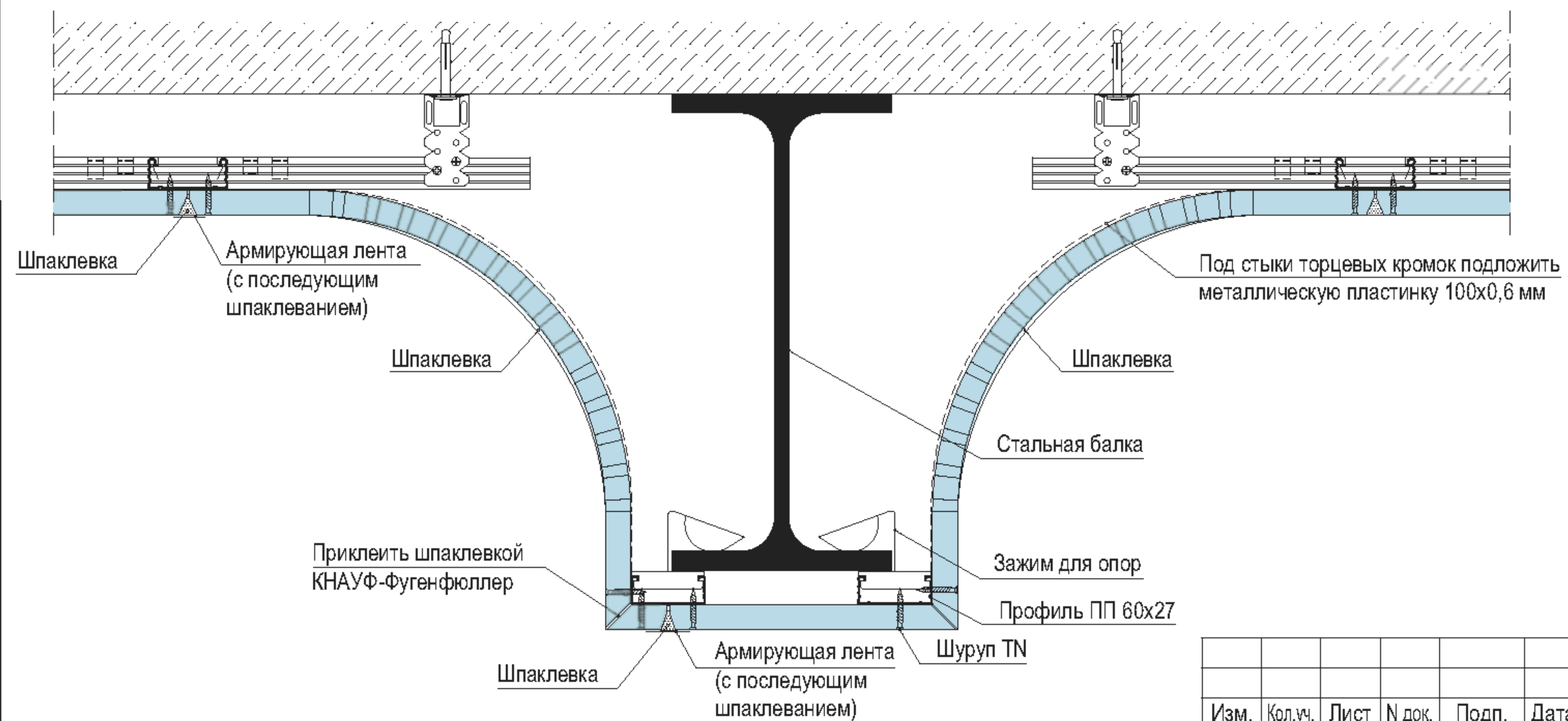
Пример применения – облицовка балки
