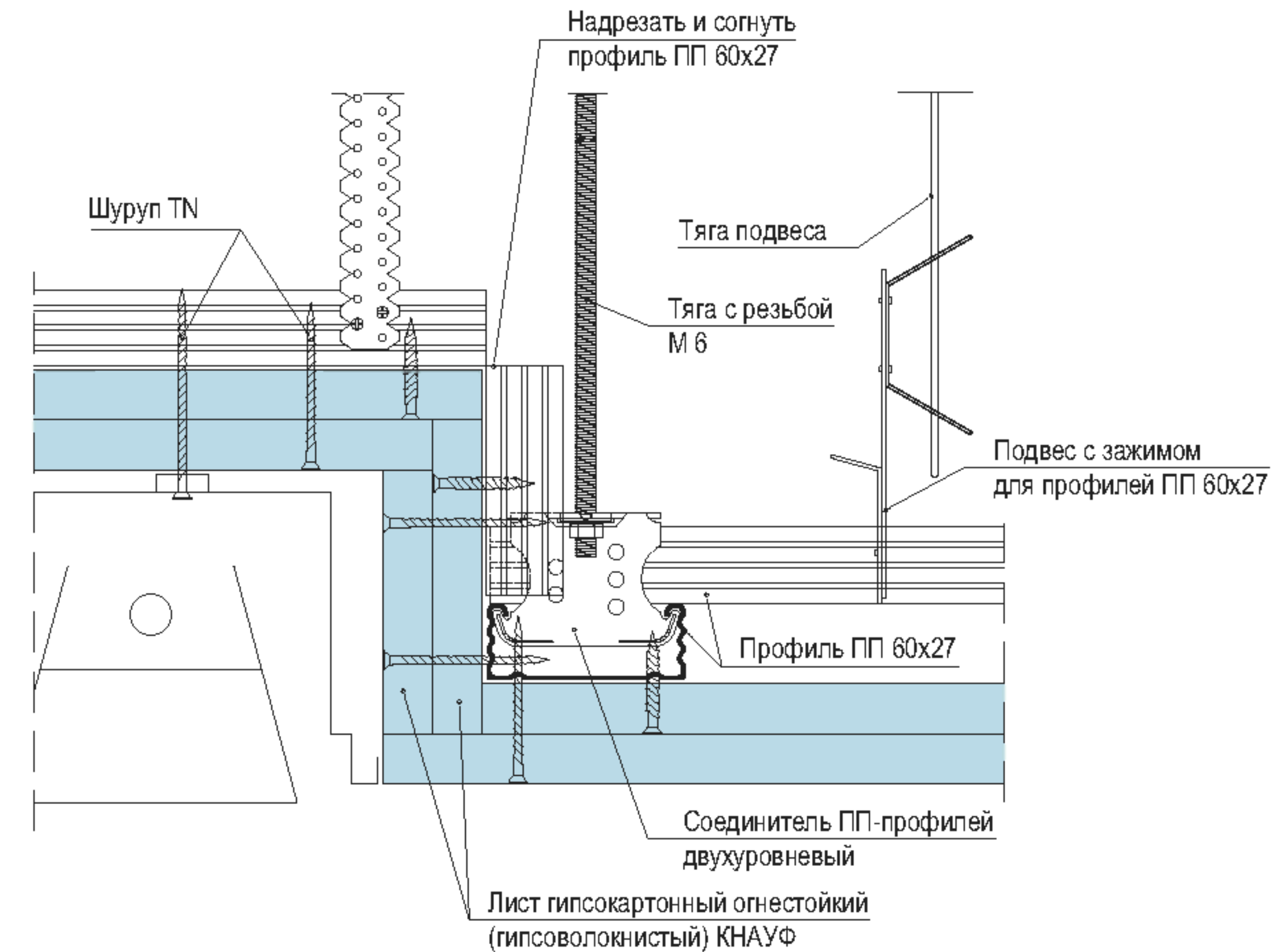
Для потолочной конструкции П112 (П212)
