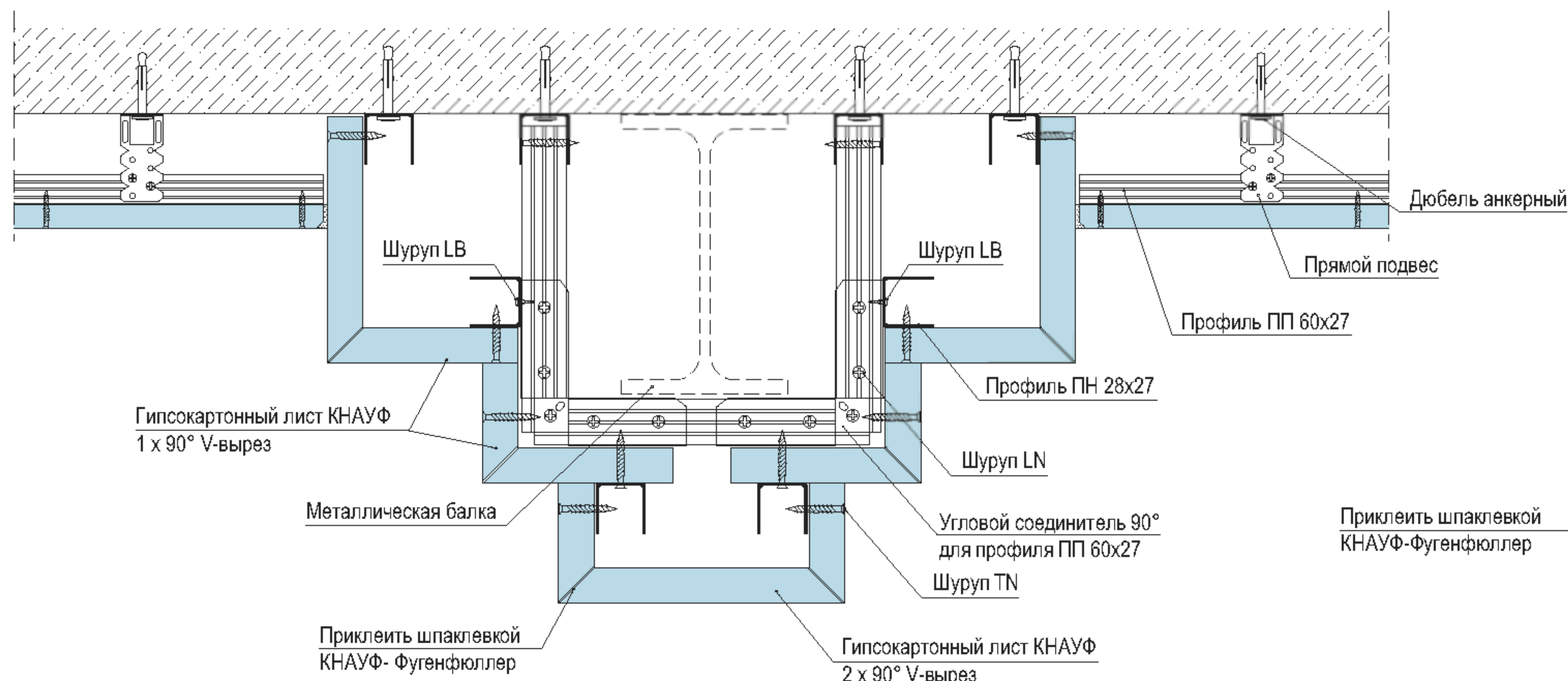
Пример применения - модульный потолок
