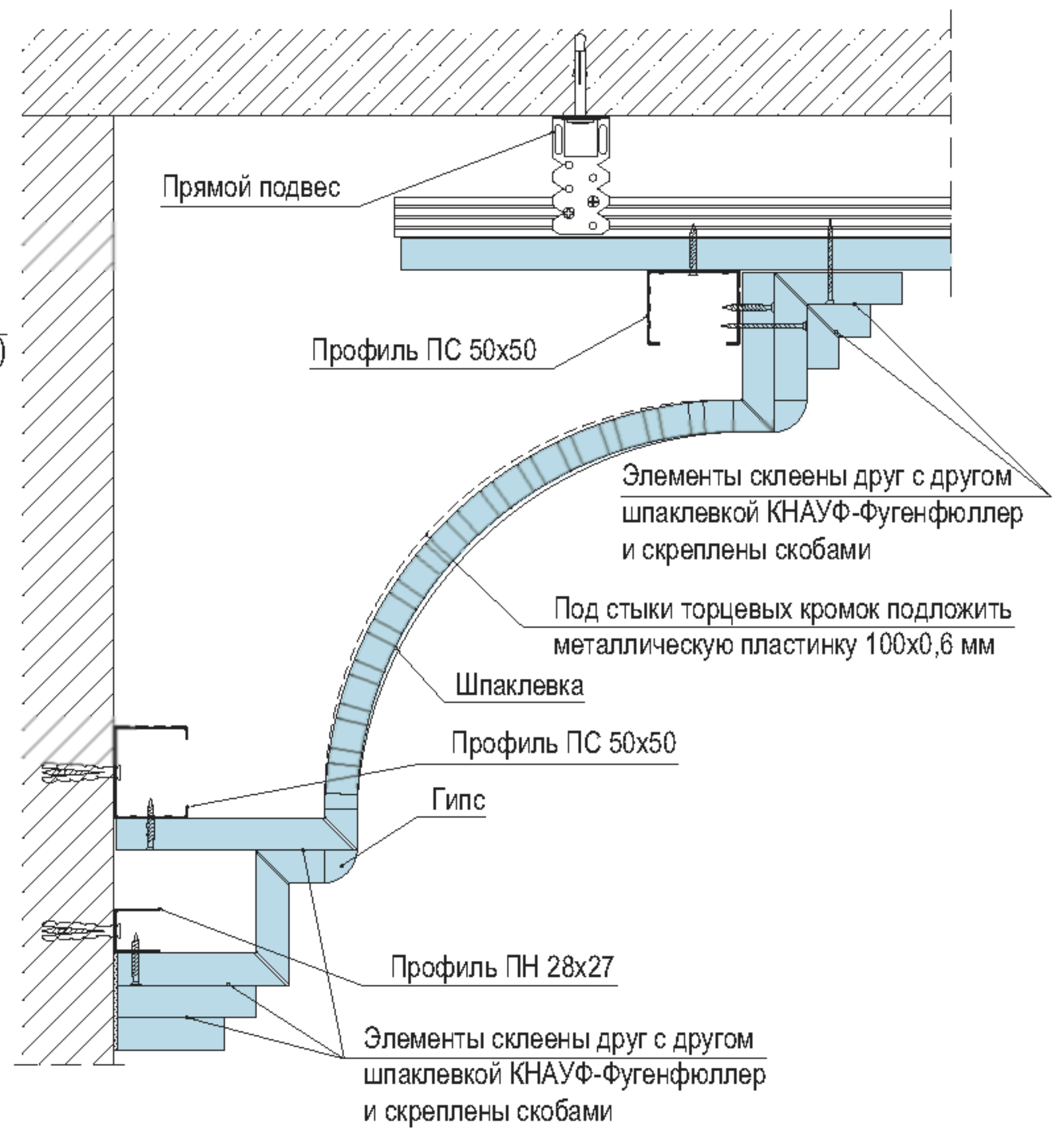
Пример применения – карниз – закругленный
