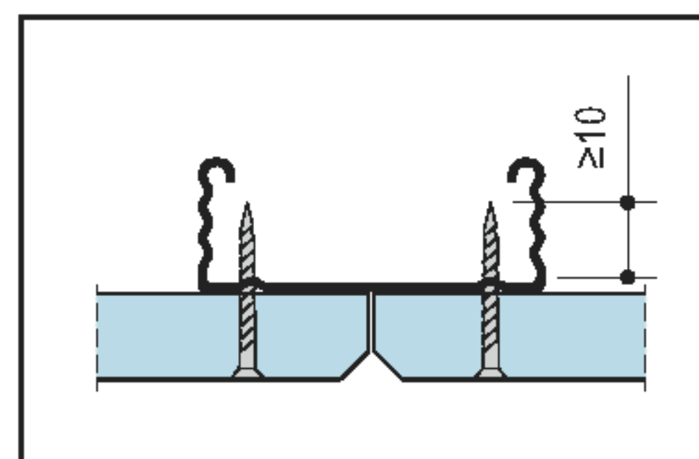
Правильное крепление к профилю гипсокартонного листа
