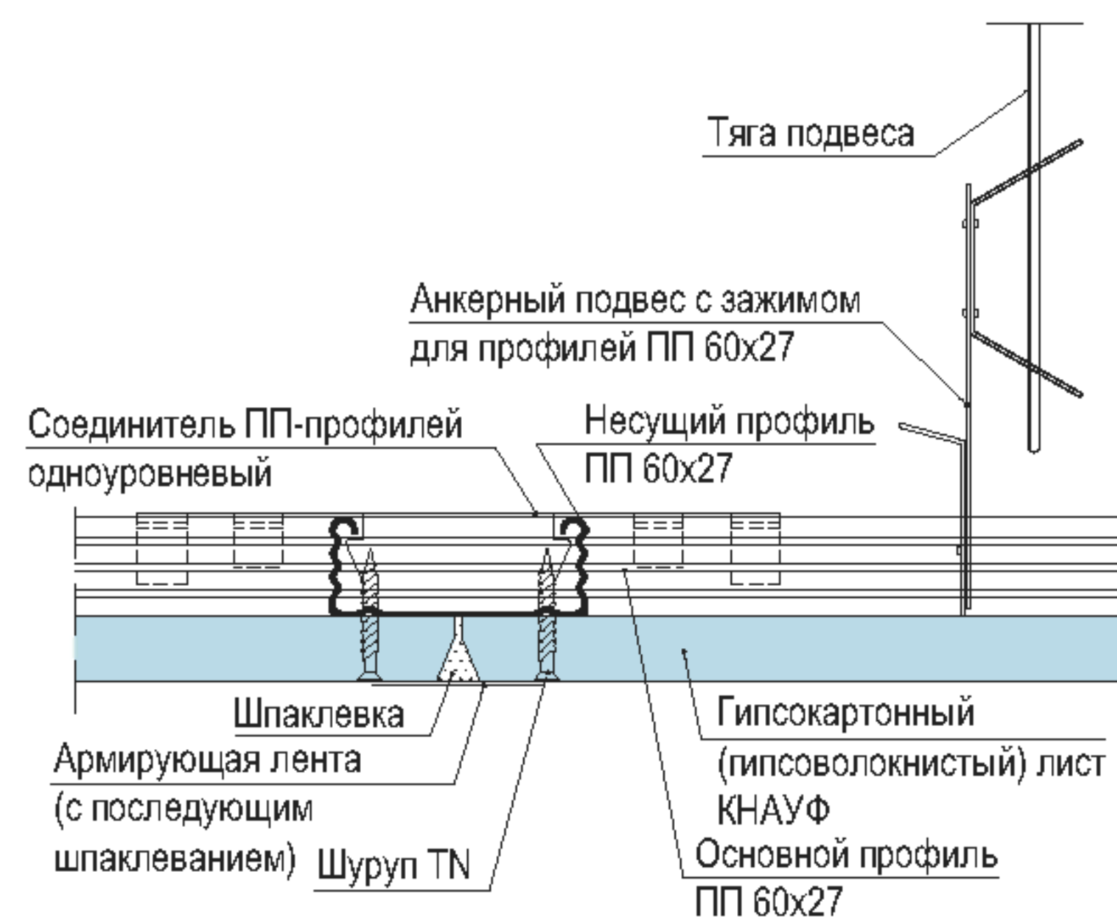
Г - Г Присоединение основных профилей
