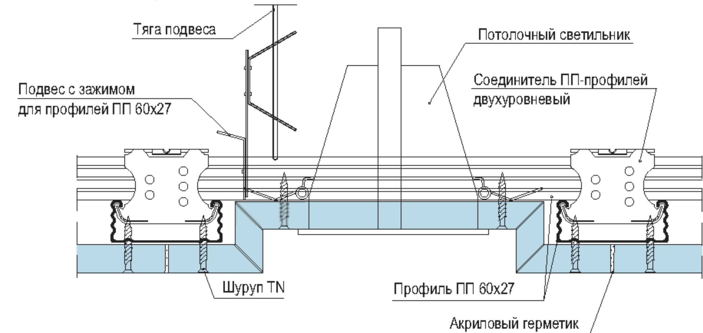
Углубление в потолке со светильником
